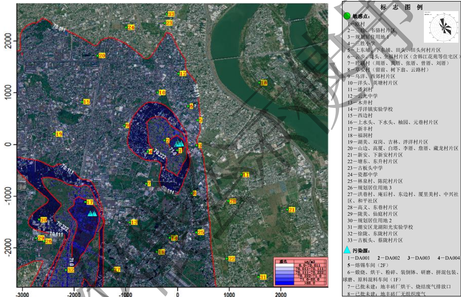
图 6.3-21 (a) 正常排放叠加现状本底浓度、在建拟建项目后 \text{PM}_{10} 日平均最大落地浓度贡献值等值线图（单位： \mu\text{g}/\text{m}^3 ）
