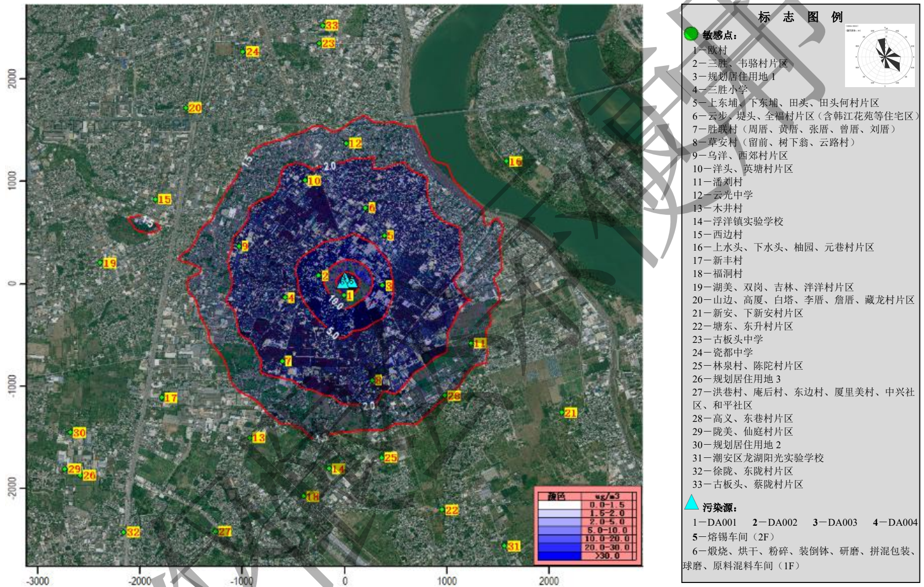
图 6.3-27 非正常排放锡及其化合物小时平均最大落地浓度贡献值等值线图（单位： \text{ug}/\text{m}^3 ）
