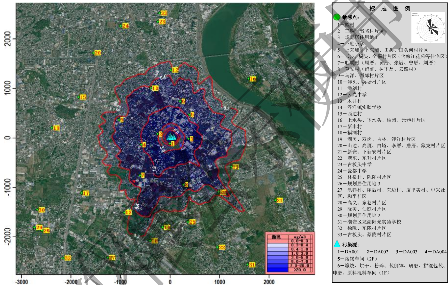
图 6.3-14 正常排放锡及其化合物 1 小时最大落地浓度贡献值等值线图（单位：ug/m³）
